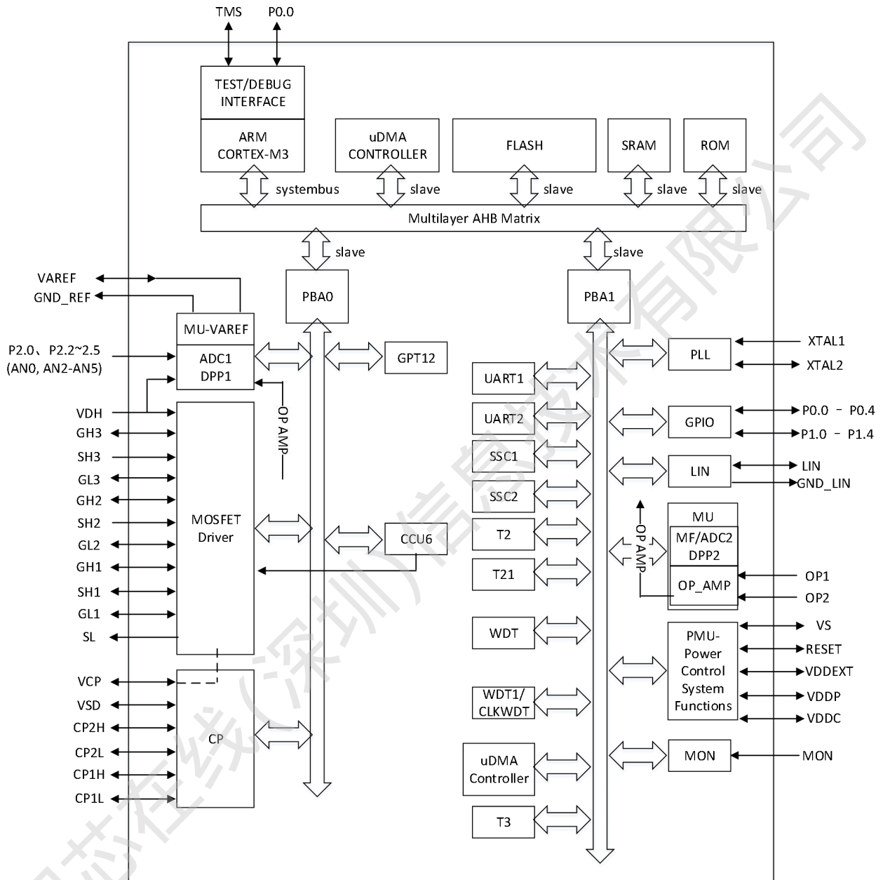
图 5-1：结构框图
