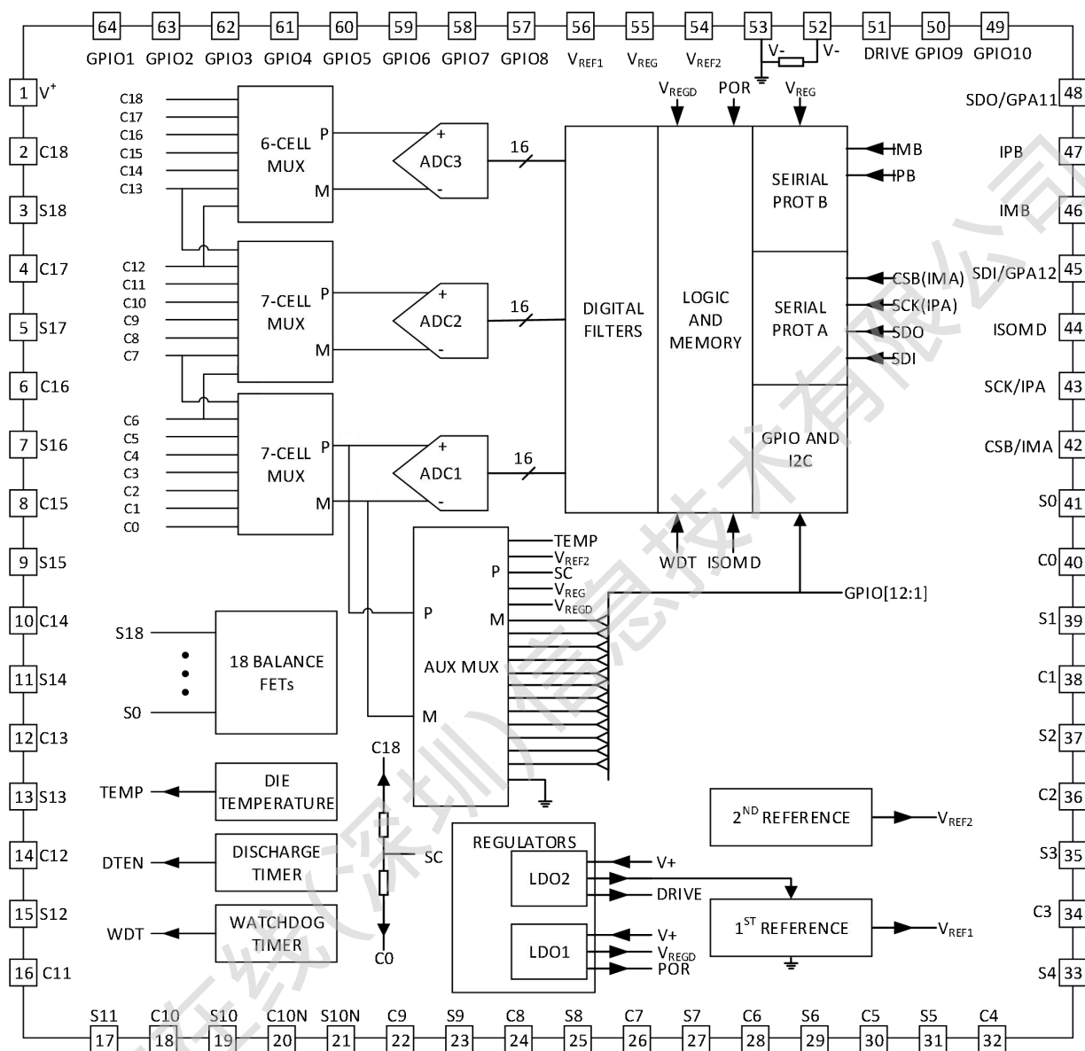
图 5-1：结构框图
