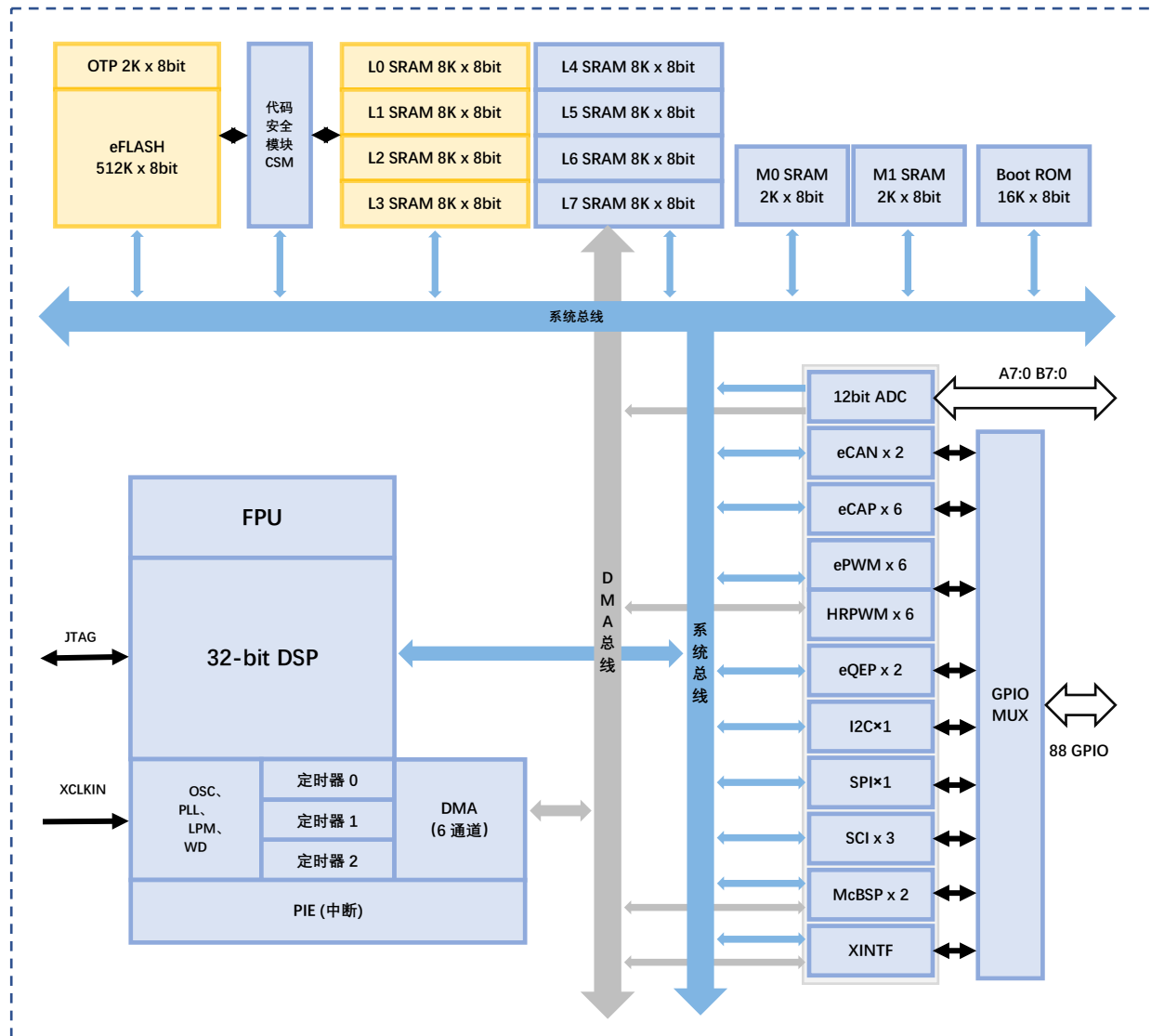
FDM320R335 的功能框图
