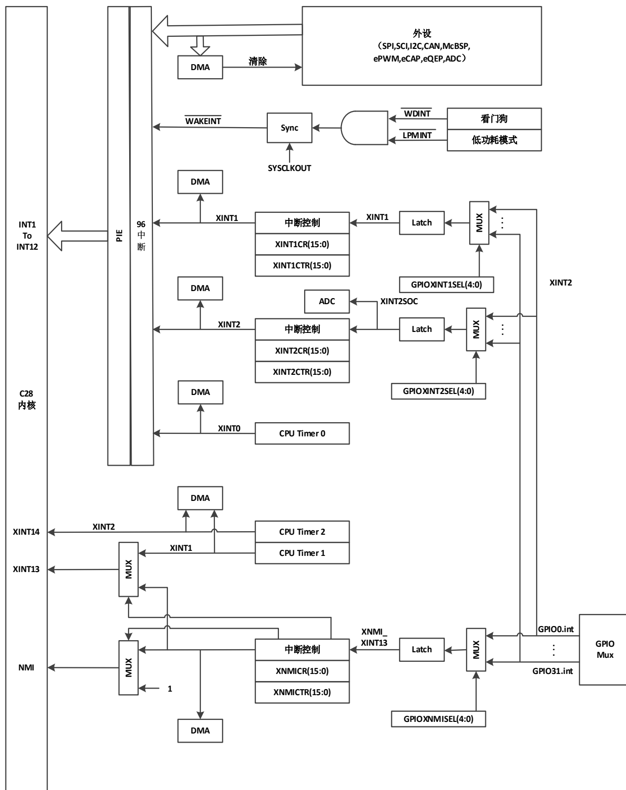
图 2. 外部和 PIE 中断源
