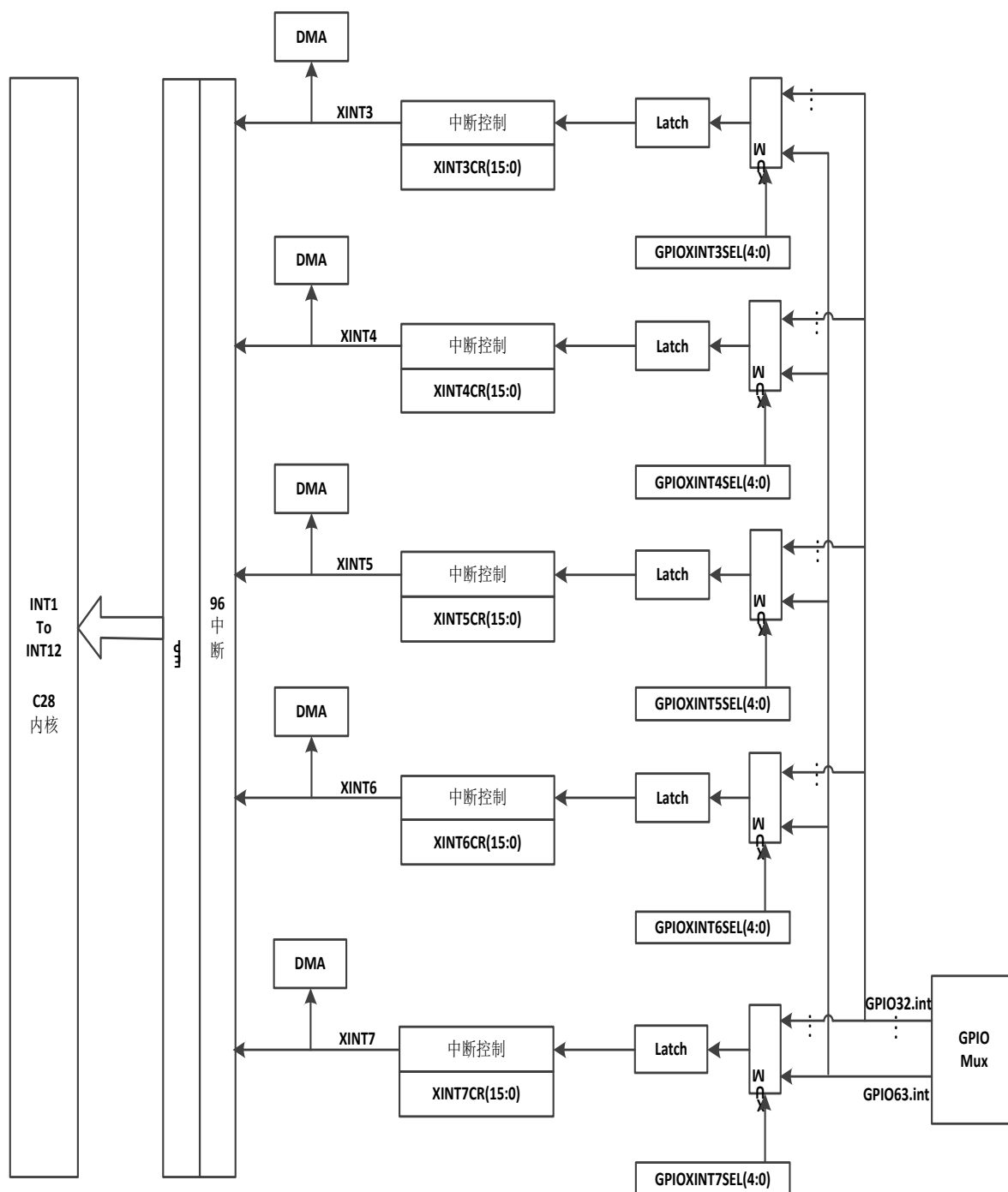
图 3. 外部中断
