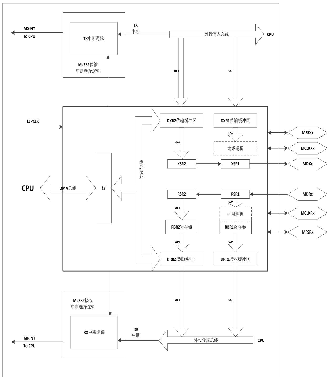
图 20. McBSP 模块
