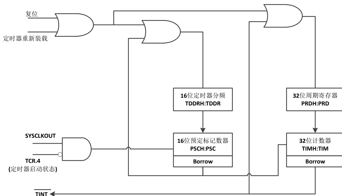
图 11. CPU 定时器
