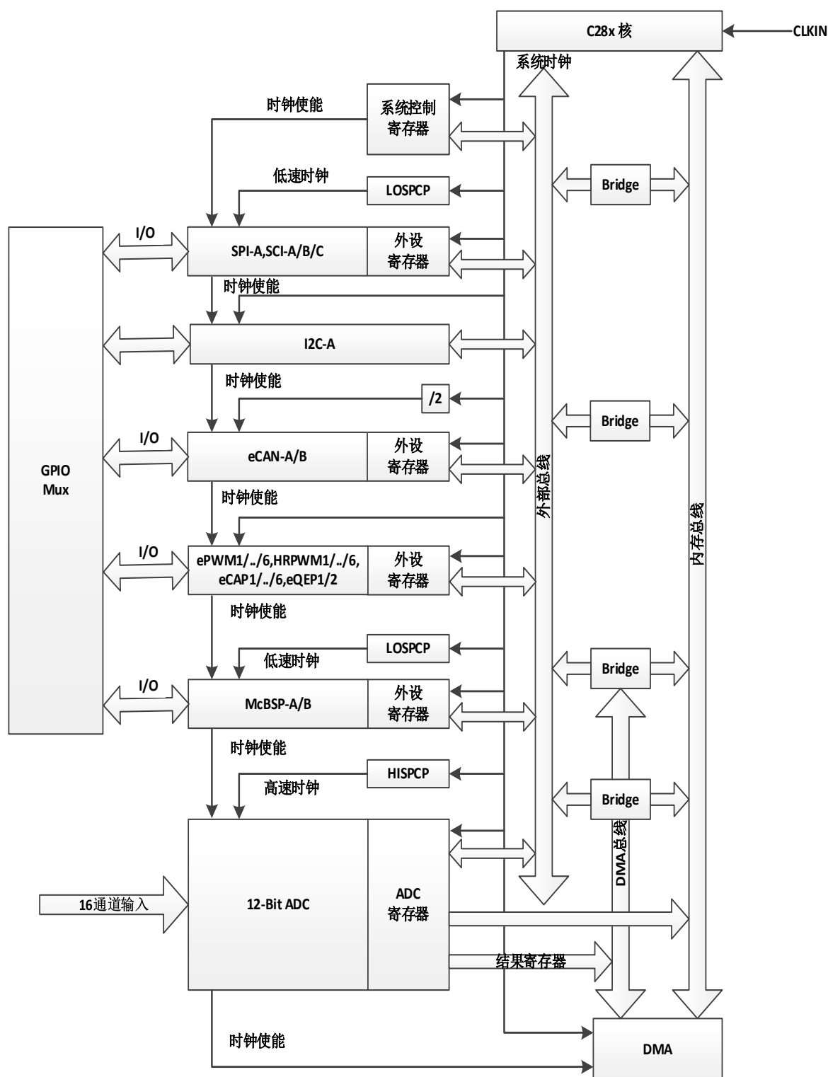
图 5.时钟与复位域
