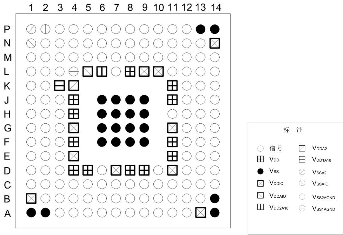
图 32. R335 176 焊球球状引脚栅格阵列(BGA)
