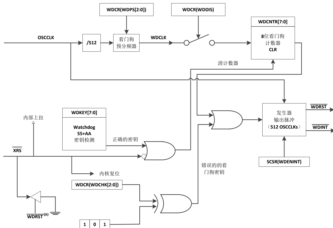
图 9. 安全装置模块
