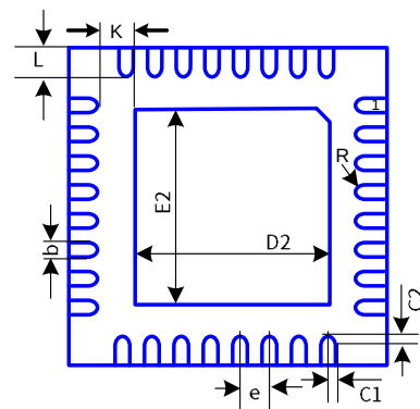
图 3-2 底视图
