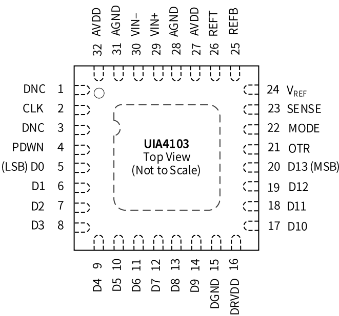
图 2-1 UIA4103 引脚配置
