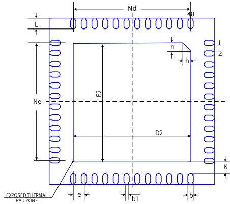
图 3-2 底视图
