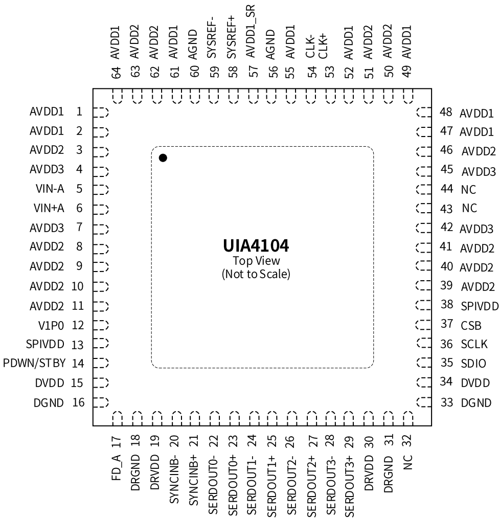
图 2-1 UIA4104 引脚配置
