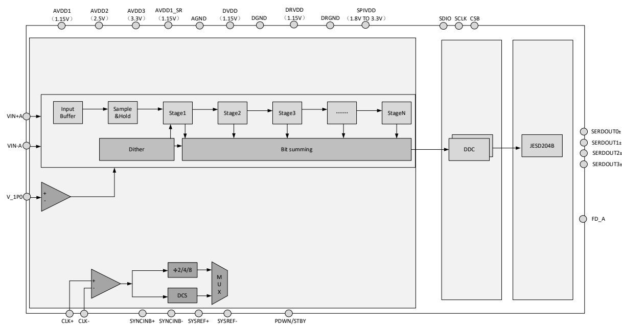
图 1-1 UIA4104 功能框图
