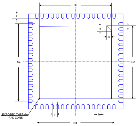
图 3-2 底视图
