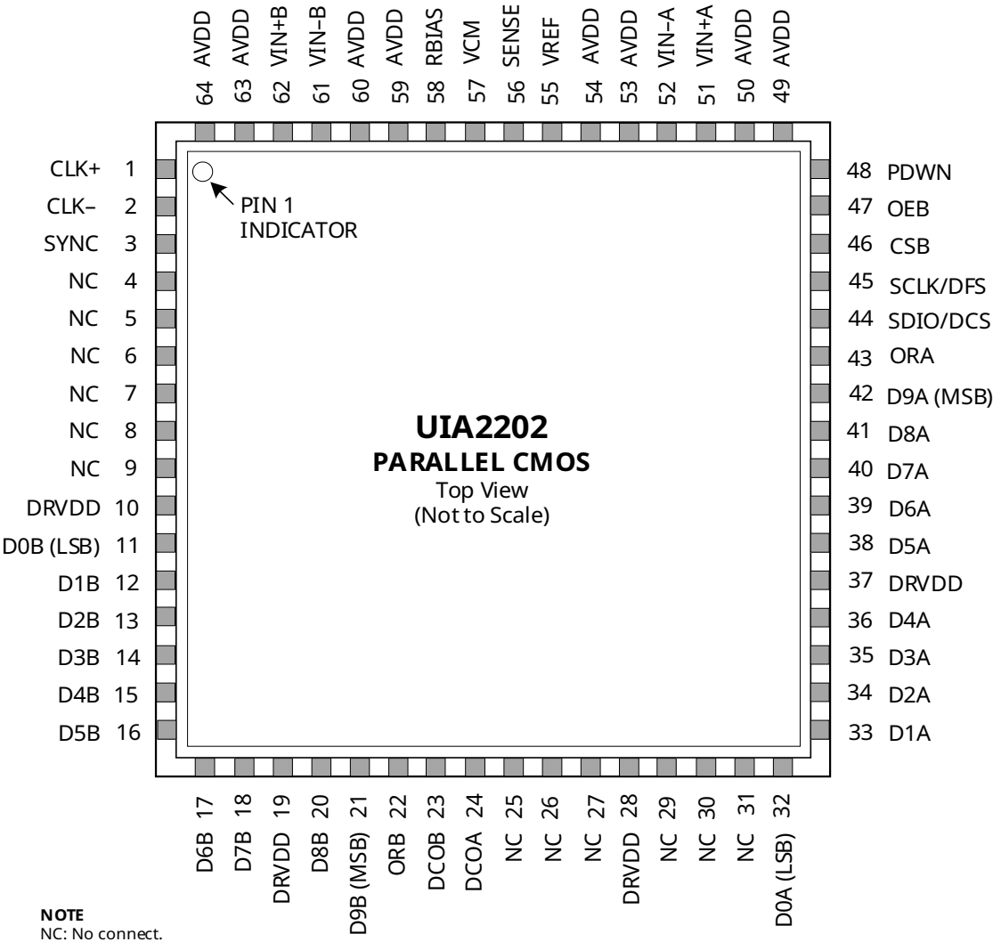
图 2-1 LFCSP 并行 CMOS 引脚配置
