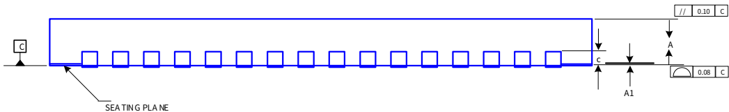
图 8-3 侧视图
