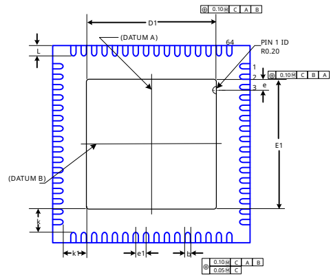
图 8-2 底视图
