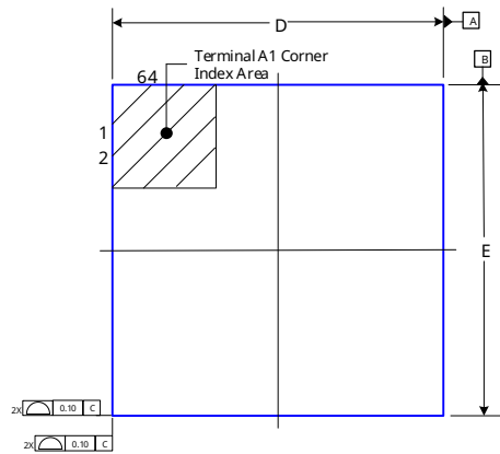
图 8-1 顶视图
