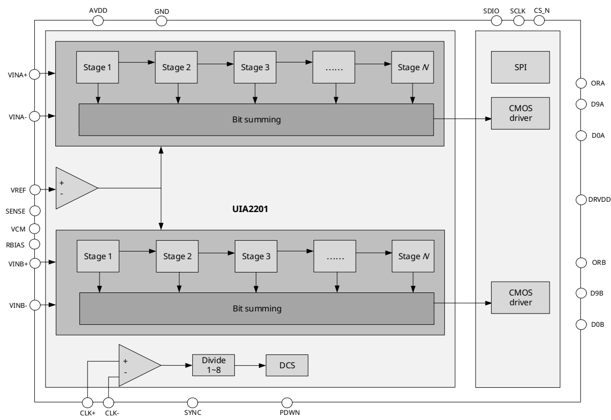
图 1-1 UIA2201 功能框图
