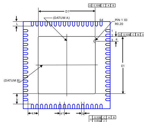
图 3-2 底视图
