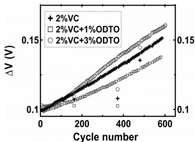
图表17 特定成分的 ODTO 电解液体系电压滞变更低
