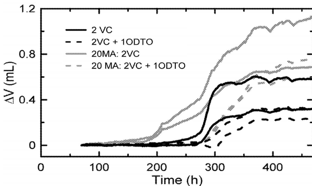
图表15 电解液中加入 ODTO 有助于抑制产气量 \Delta V
