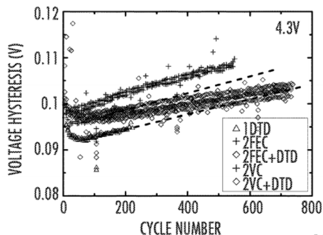
图表14 含 DTD 电解液体系拥有更小的电压滞变
