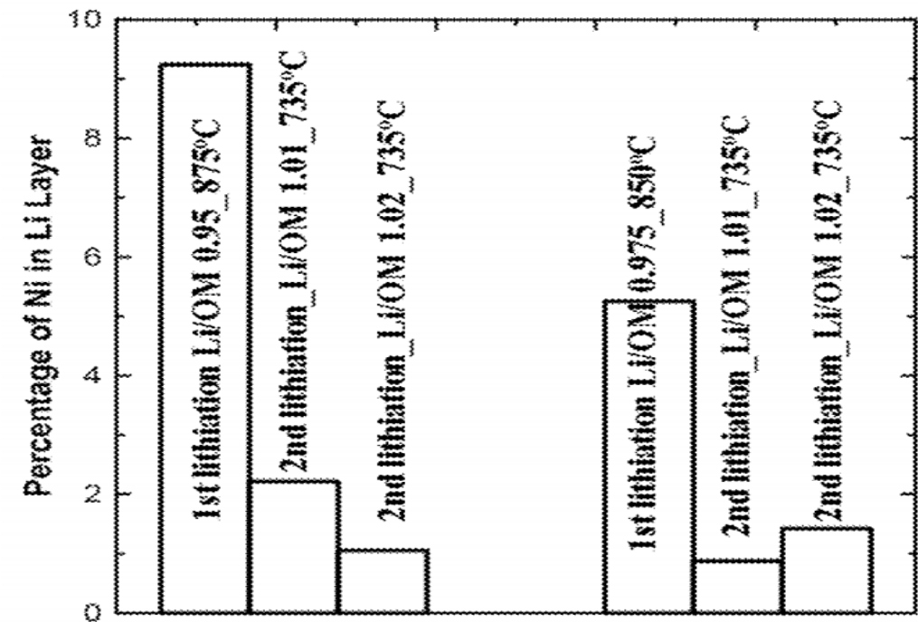
图表10 新工艺经过二次锂化反应，锂镍混排程度大幅降低
