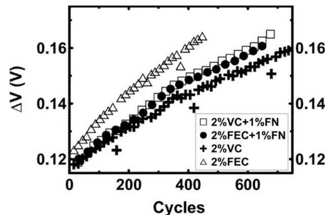
图表21 松下 1030 体系中 FN 没有减小电压滞变
